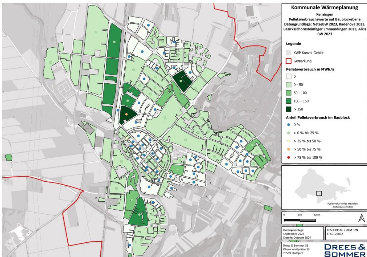
Abbildung 36: Pelletsverbrauch mit prozentualem Anteil am Baublock (Ausschnitt Kenzingen)
