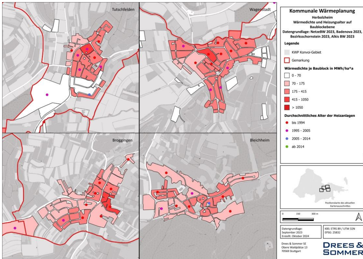
Abbildung 12: Wärmedichten (MWh/ha*a) und durchschnittliches Heizungsalter auf Baublockebene für Teilorte Herbolzheim
