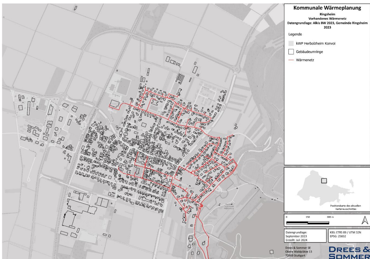
Abbildung 24: Wärmenetzinfrastruktur in Ringsheim
